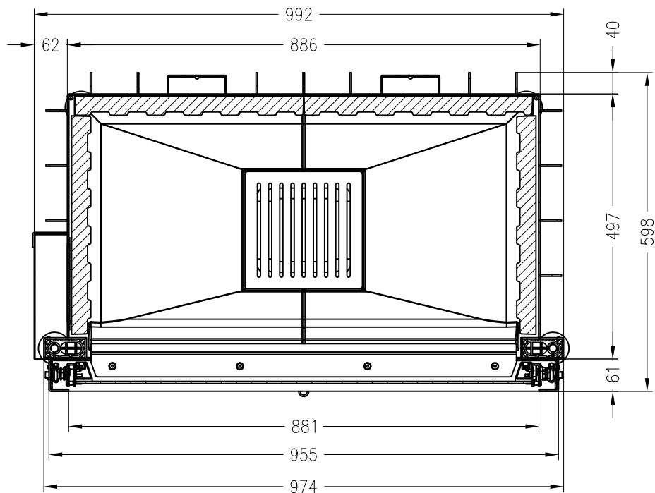
Horizontalschnitt M~1:10
